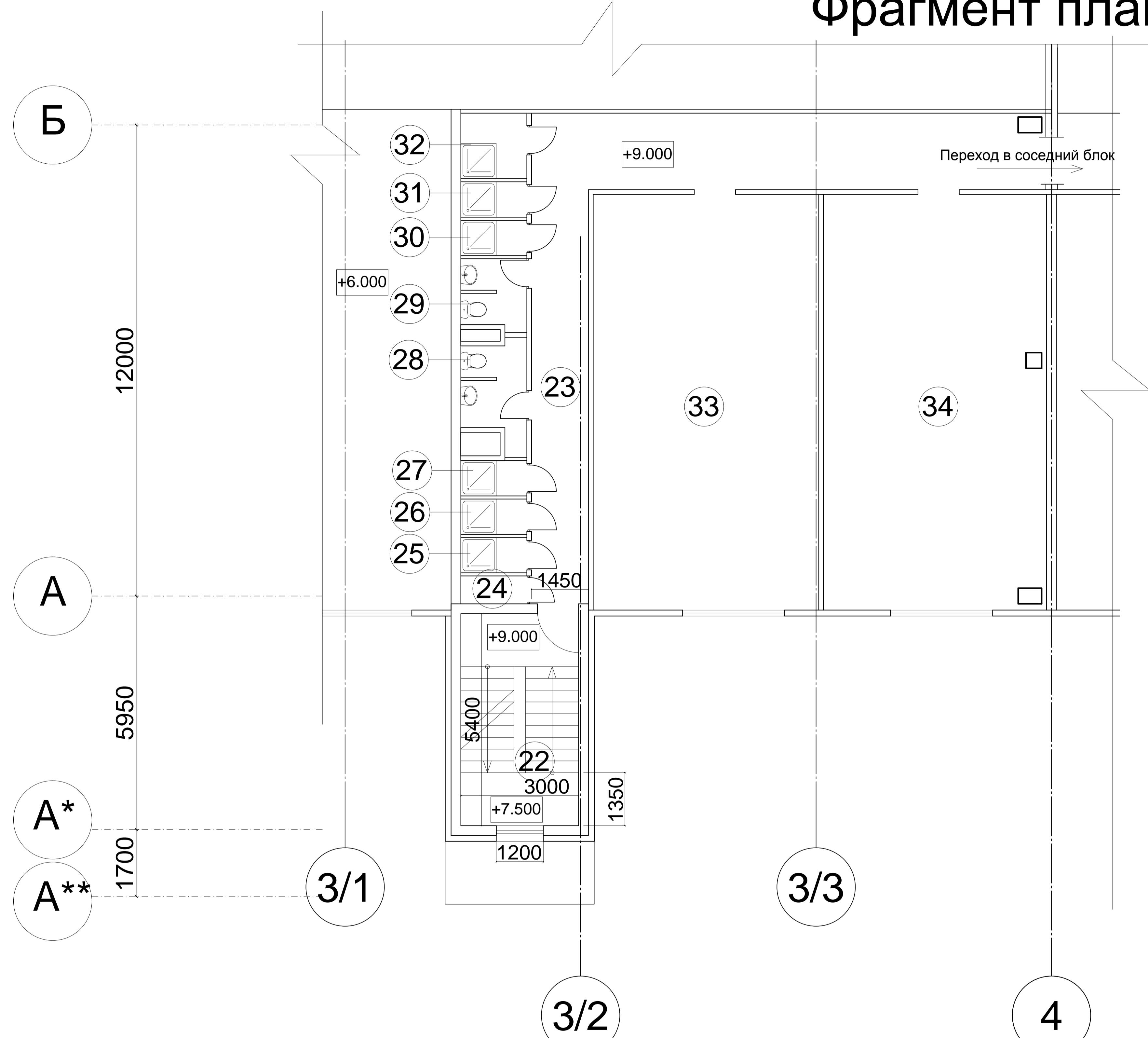
ЭКСПЛИКАЦИЯ ПОМЕЩЕНИЙ НА ОТМ. +9.000 секции №4
